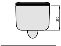
Wc Brio sospeso Wc Brio wall-hung Bidet Brio sospeso Bidet Brio wall-hung
