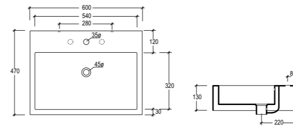
cod. QULAV60 Lavabo Quad monoforo cm. 60 appoggio o sospeso (senza foro o tre fori su richiesta) Countertop or wall-hung washbasin Quad one hole cm 60 (without hole or three holes on request)
