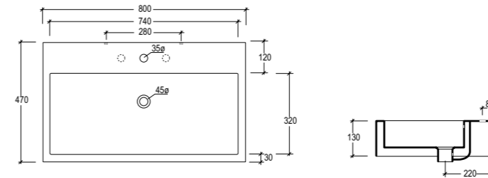
cod. QULAV80 Lavabo Quad monoforo cm. 80 appoggio o sospeso (senza foro o tre fori su richiesta) Countertop or wall-hung washbasin Quad one hole cm 80 (without hole or three holes on request)
